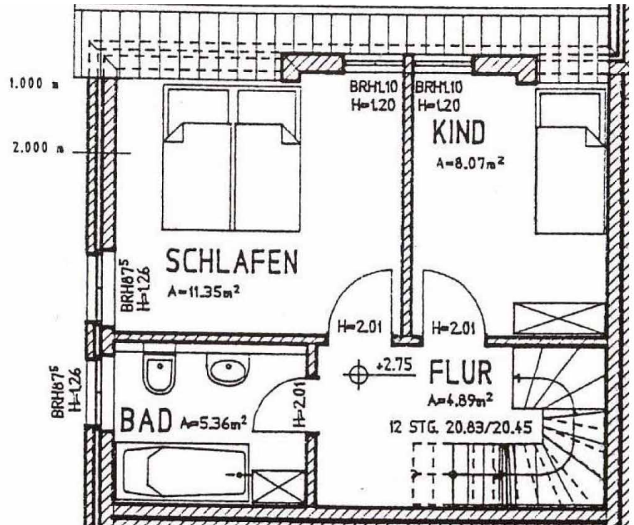
Grundriss Obergeschoss
