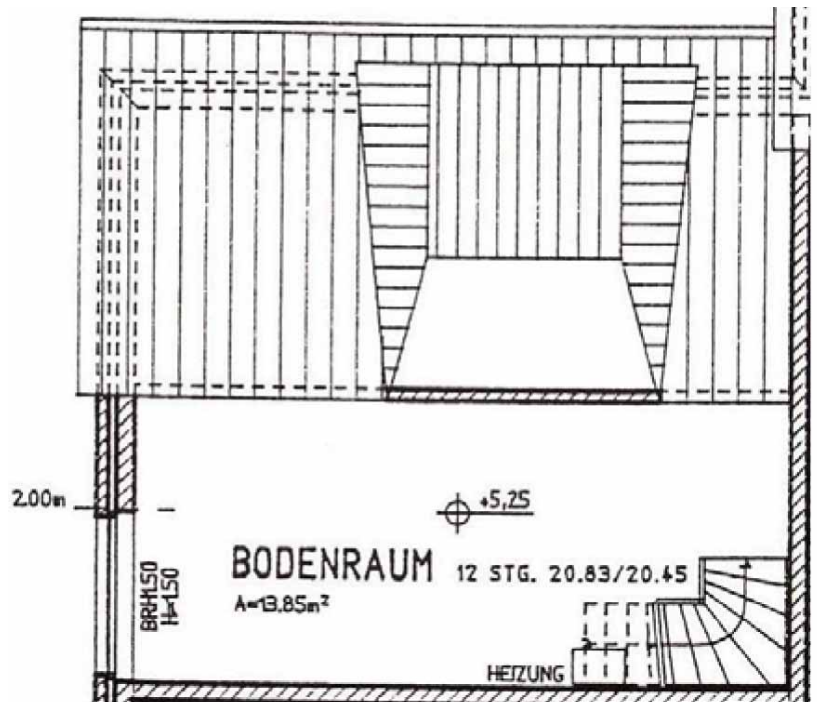
Grundriss Spitzboden
